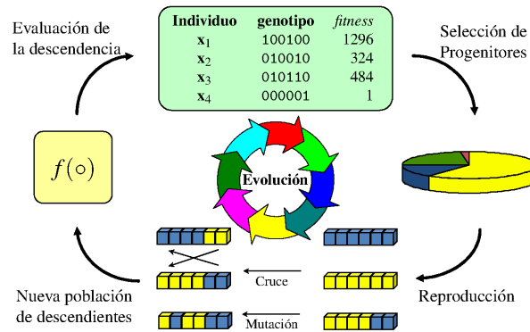
Figura 2.3: Diagrama de flujo del ciclo evolutivo de un algoritmo genético. Tomada de [50].
