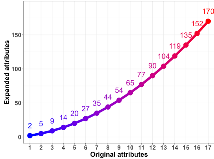
Figura 2.2: Crecimiento del número de atributos bajo una expansión polinomial de grado 2 sin término de sesgo. Fuente: Elaboración propia.
